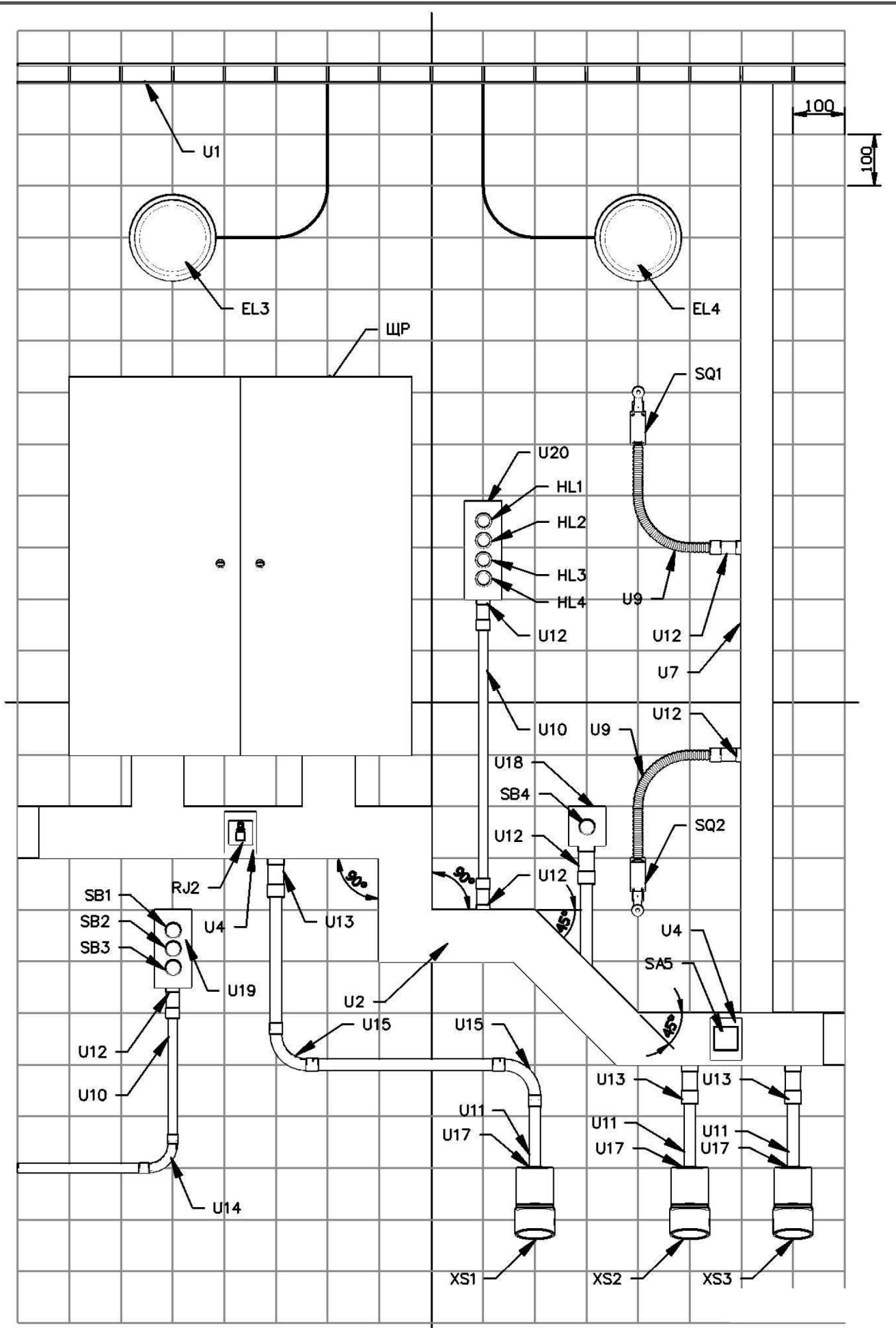
Монтажная схема вид "Б"
