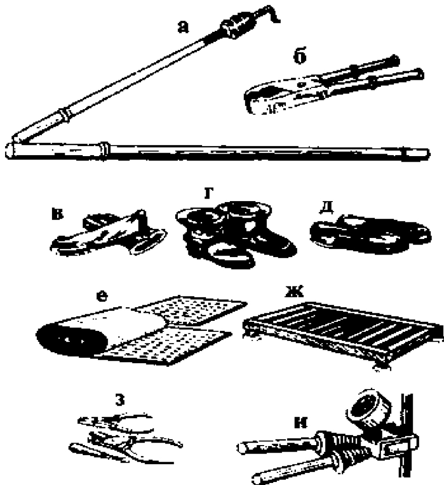
Рисунок 2 - Защитные средства, применяемые при обслуживании электроустановок: а — изолирующие штанги; б — изолирующие клещи; в — диэлектрические перчатки; г — диэлектрические боты; д — диэлектрические галоши; е — резиновые коврики и дорожки; ж — изолирующая подставка; з — монтерские инструменты с изолирующими ручками; и — токоизмерительные клещи; к — указатель напряжения
