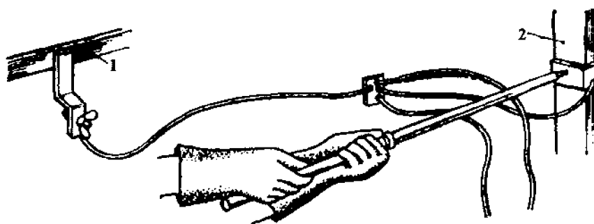
Рисунок 1- Временное переносное заземляющее устройство: 1 — шина сети заземления; 2 — токоведущая часть электроустановки
