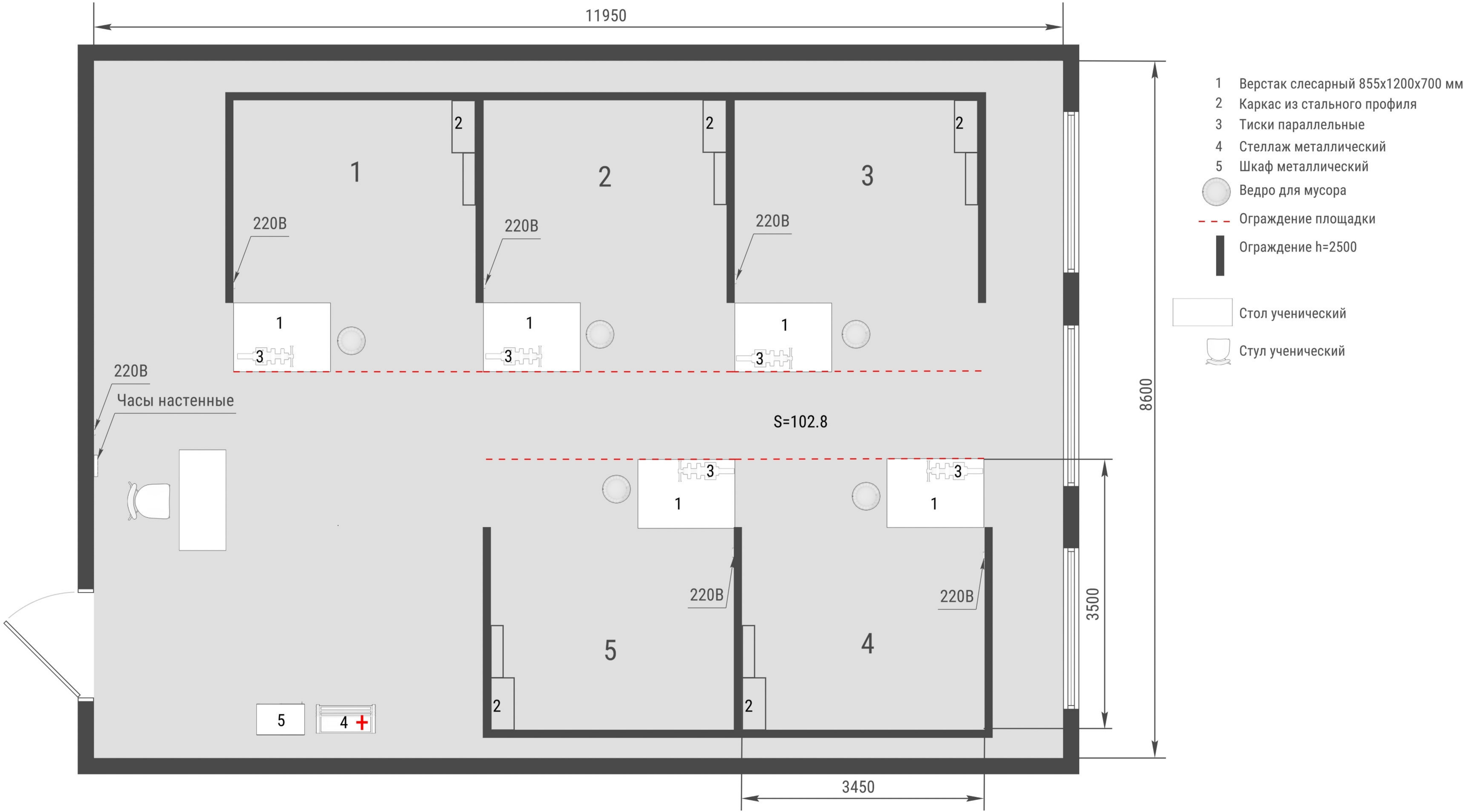
План застройки конкурсной площадки по компетенции "Сантехника и отопление" на 5 рабочих мест
