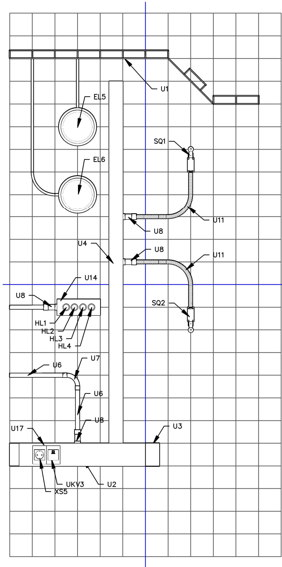
Монтажная схема вид "В"
