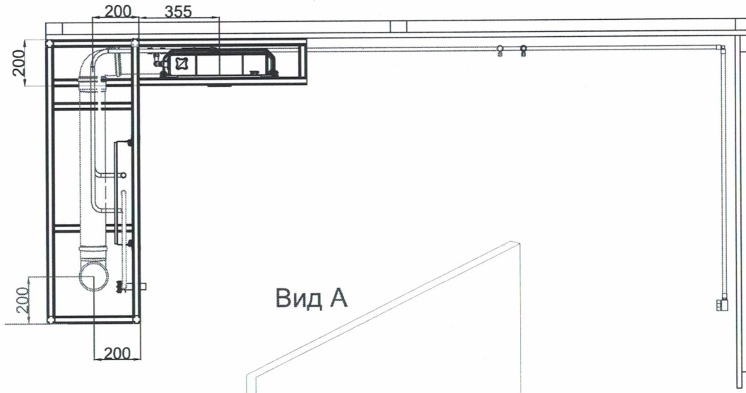
ВИД Сверху
