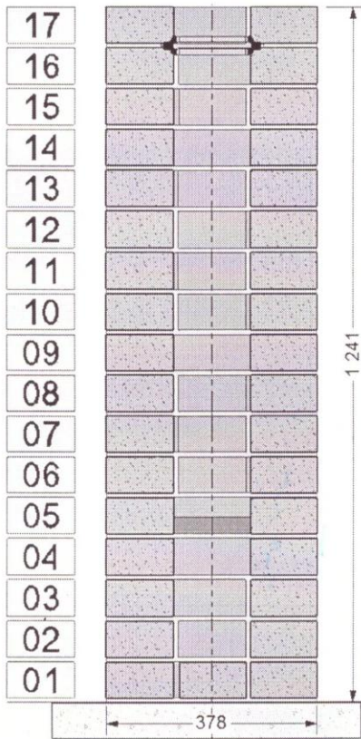
Разрез сбоку
