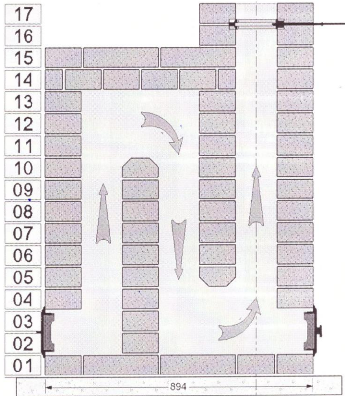
Разрез спереди
